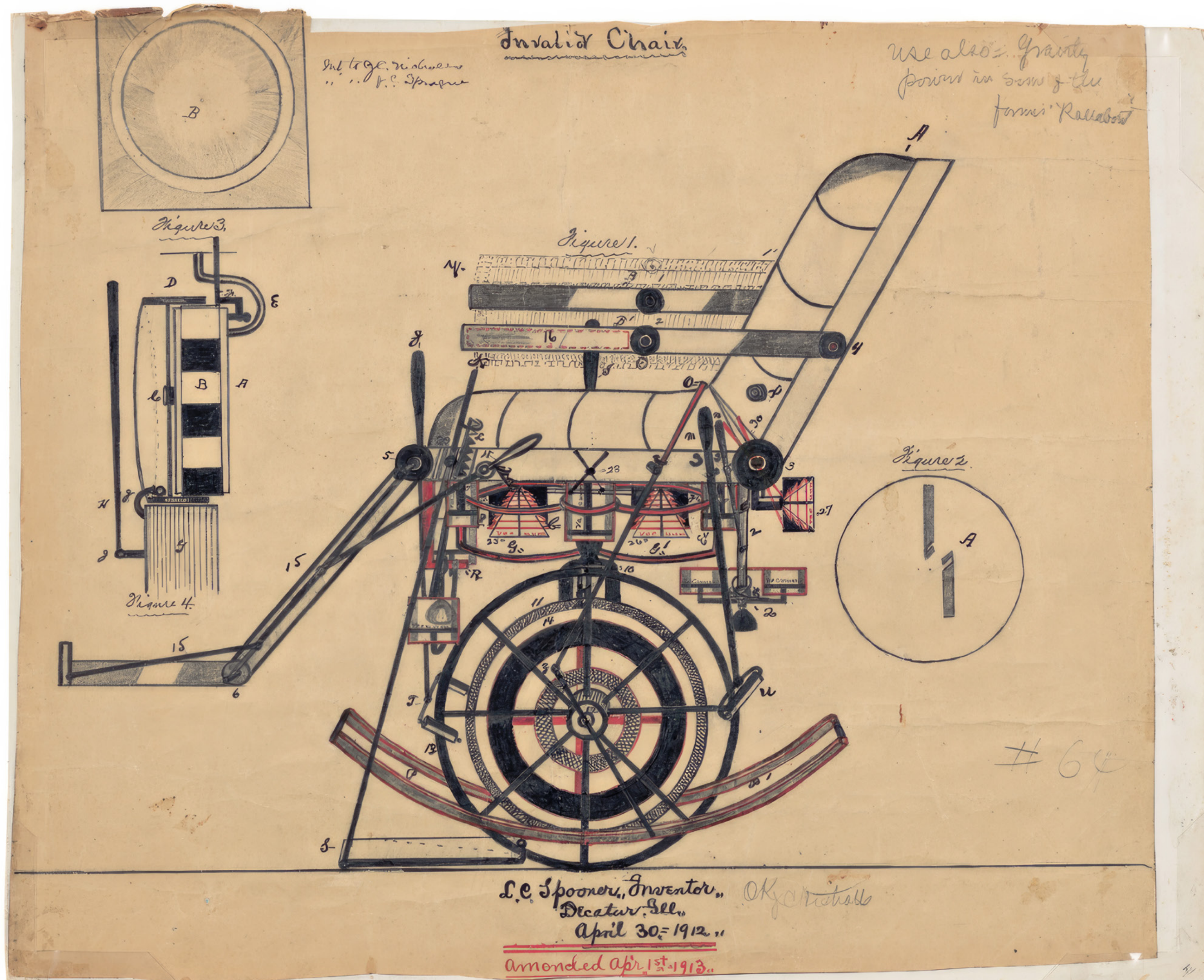
L.C. Spooner Invalid Chair, 30 avril 1912, encre et mine graphite sur papier collé sur carton, 38 x 47,5 cm
