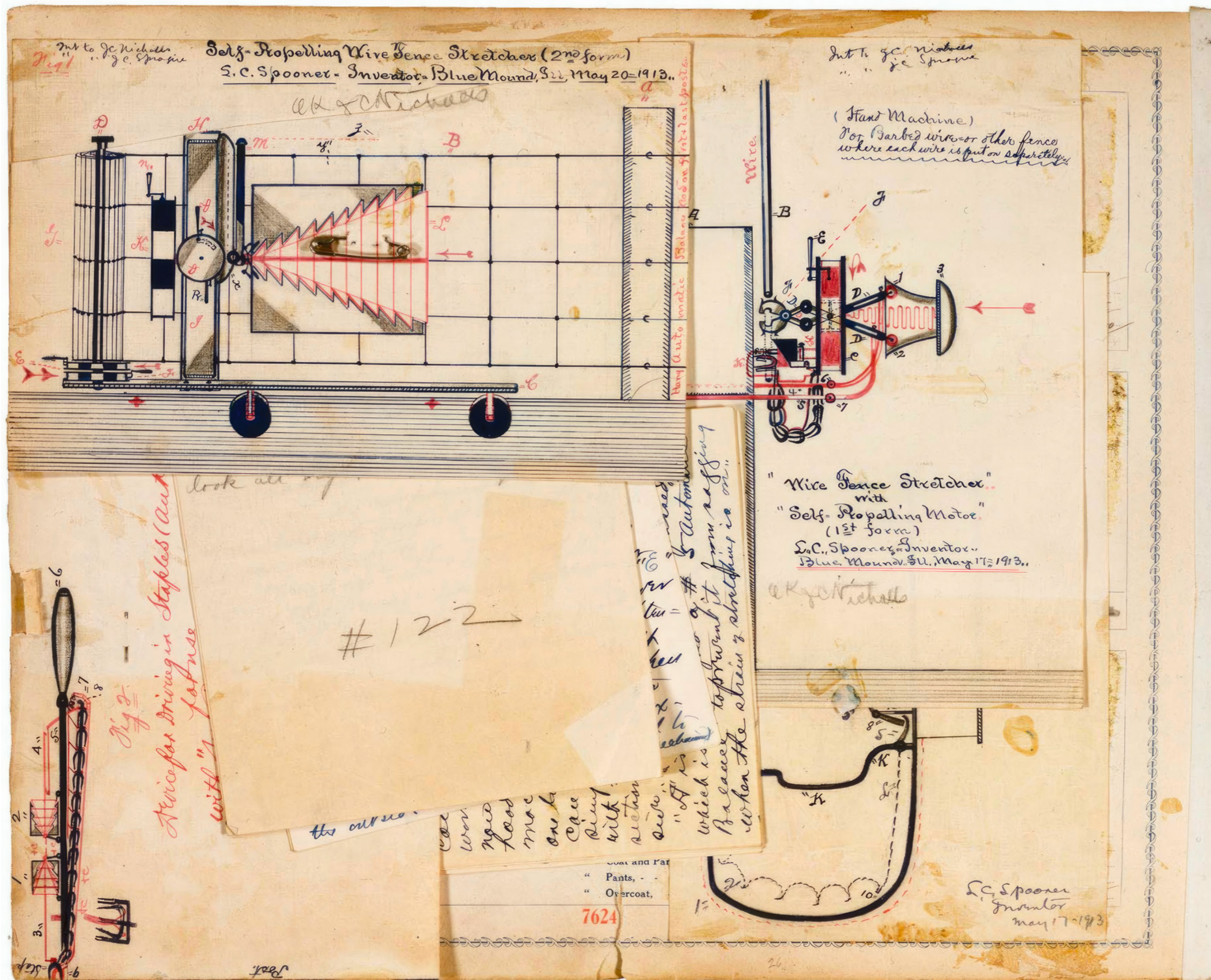
L.C. Spooner Self-Propelling Wire Fence Stretcher, 20 mai 1913, encre bleue, encre rouge, mine graphite, épingle à nourrice, aiguille et papier collé sur carton, 38 × 47,5 cm
